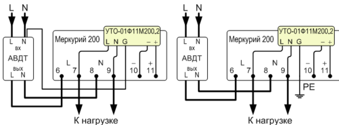
Рис. 1 Схемы подключения устройства «УТО-01Ф11М200.2» с АВДТ до счетчика.
