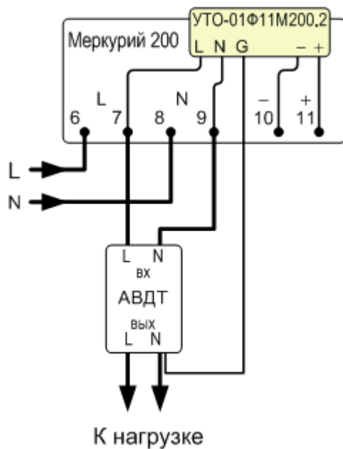
Рис. 2 Схема подключения устройства «УТО-01Ф11М200.2» с АВДТ после счетчика.
