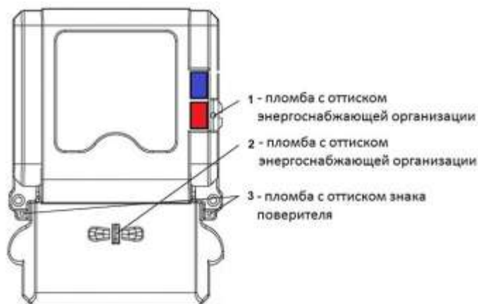
Рис.6 – Схема пломбирования УТО-01Φ101.
