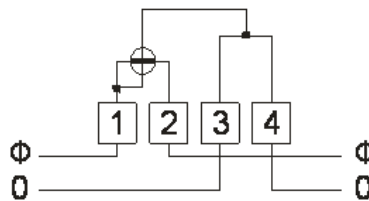
Рис. 5 – Схема подключения УТО-01Φ101:
