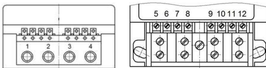
Рис. 2 - Клеммная колодка УТО-01Ф101, 1,3 - зажимы проводов со стороны сети; 2, 4 - зажимы проводов со стороны потребителя.
